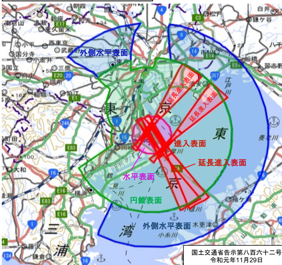
東京国際空港周辺の制限表面図
